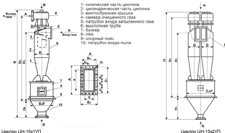
Циклон ЦН-15х1УП
